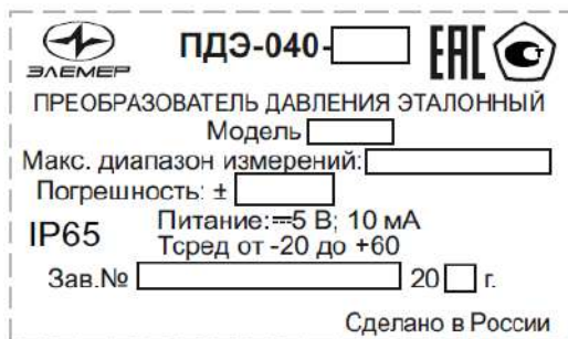
Рисунок А.4 – Табличка с маркировкой ПДЭ-040
